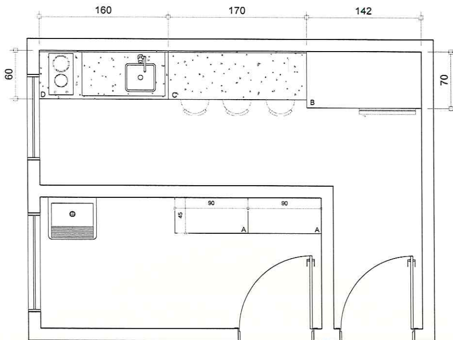
Planta Baixa
