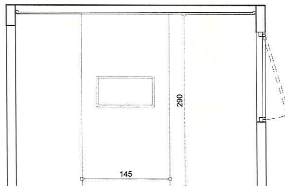
Elevação Painel TV
