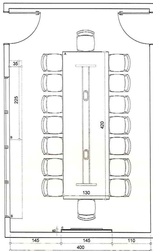
Planta Baixa
