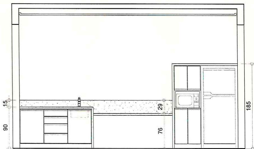
Elevação Cozinha
