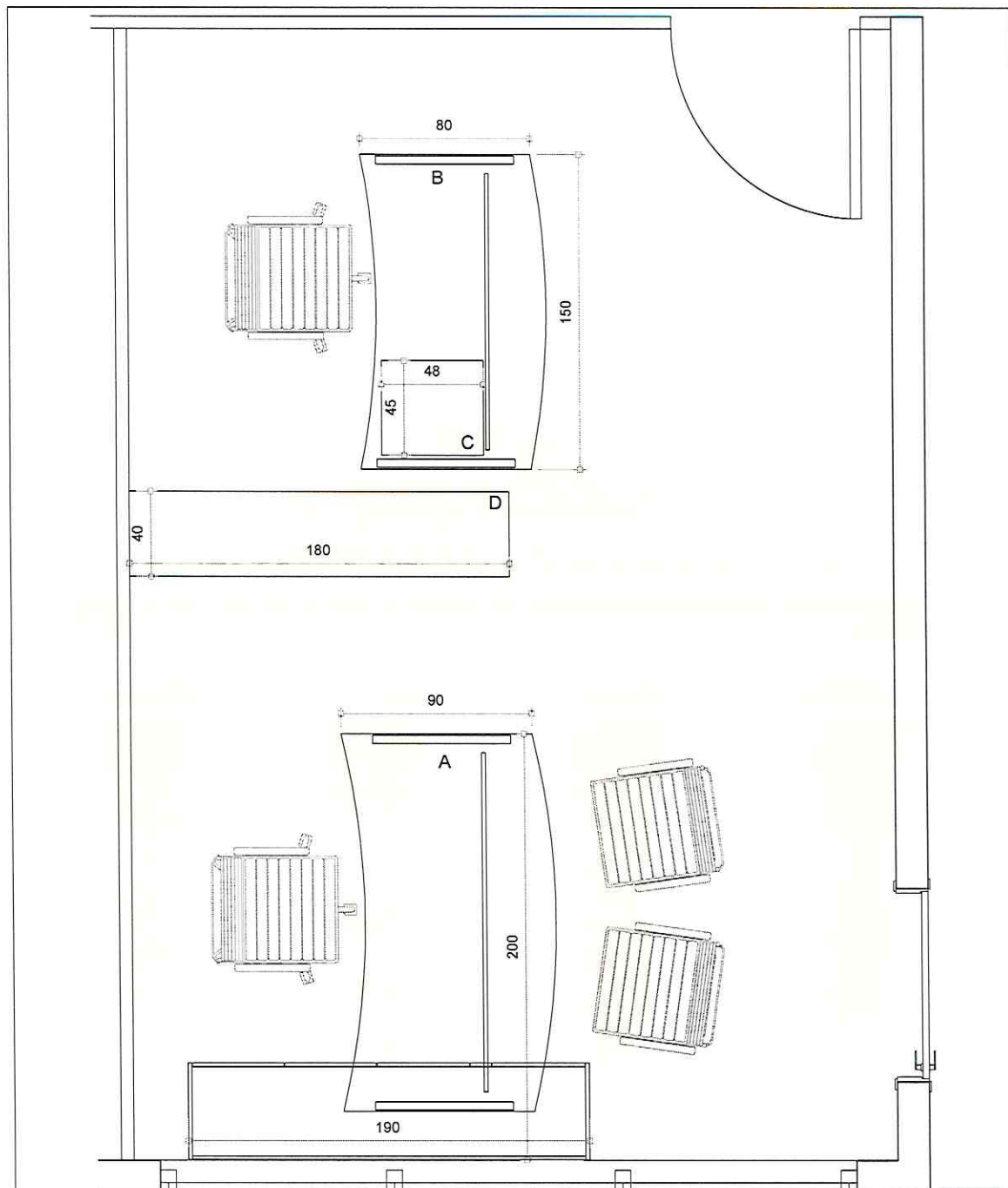
Planta Baixa Escala 1:25
